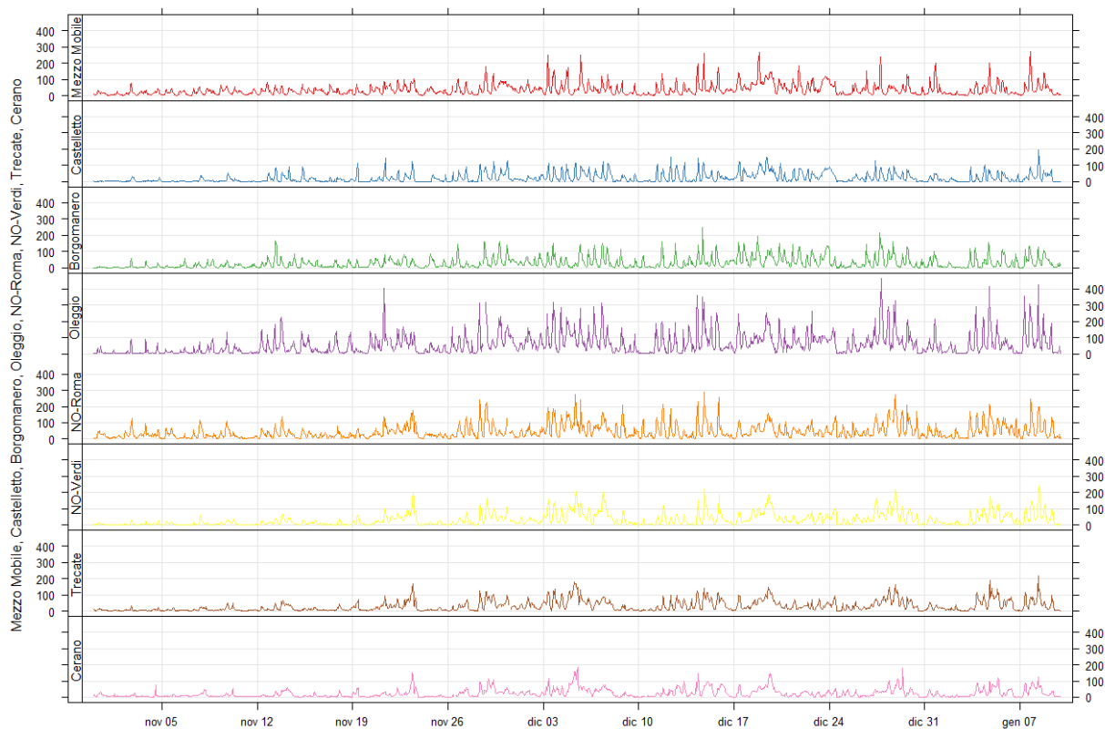
Figura 21: confronto delle medie orarie di Monossido di Azoto
