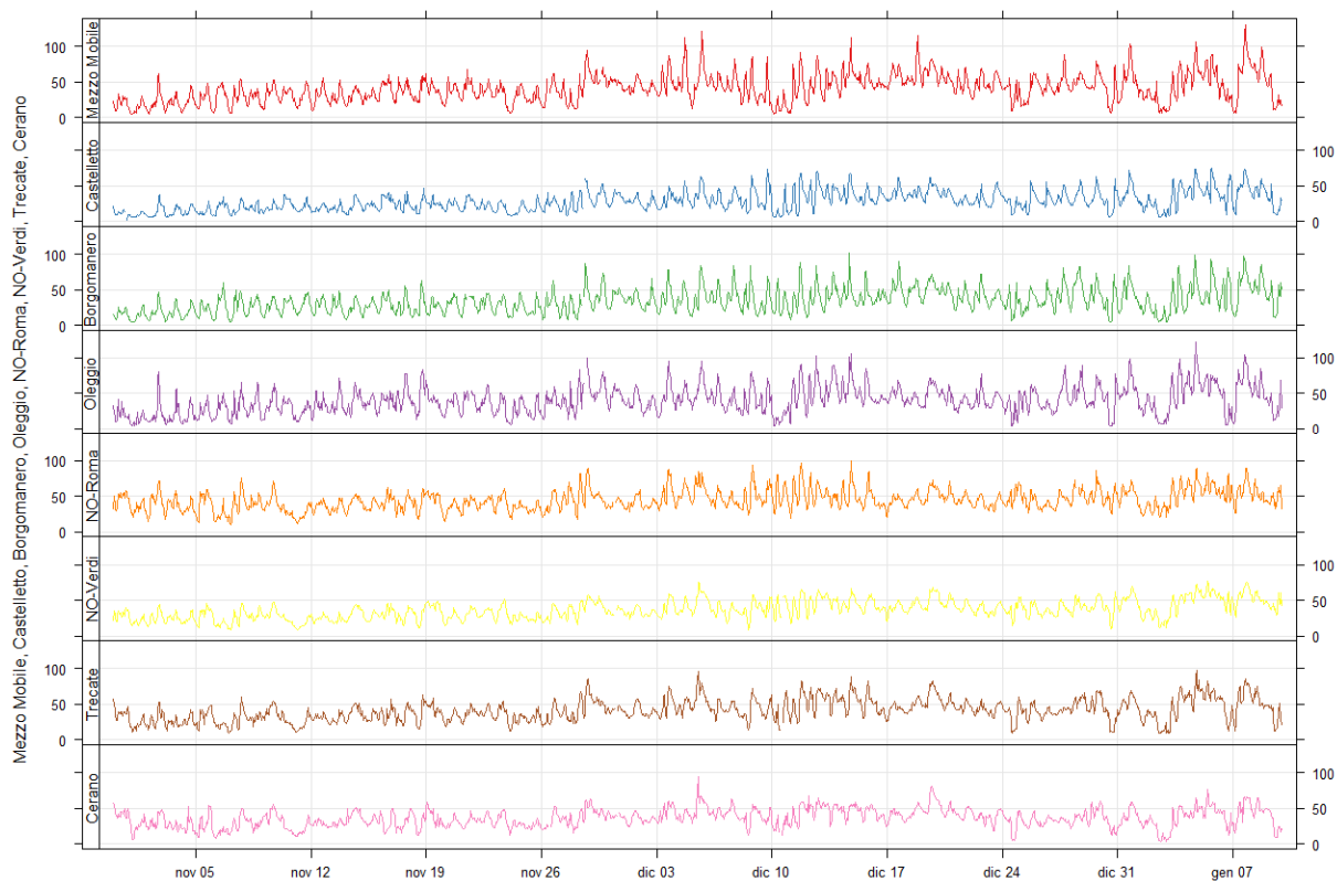
Figura 14: confronto delle medie orarie di Biossido di Azoto
