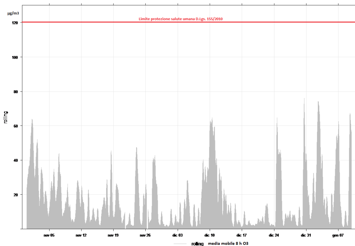
Figura 28: medie mobili otto ore Ozono
