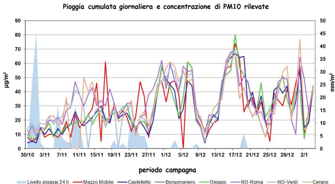
Figura 50: pioggia cumulata giornaliera e concentrazione di PM10 rilevata nelle stazioni di interesse
