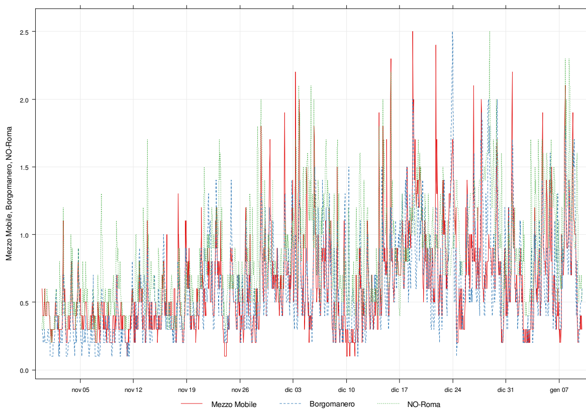
Figura 34: confronto delle medie orarie di Monossido di Carbonio
