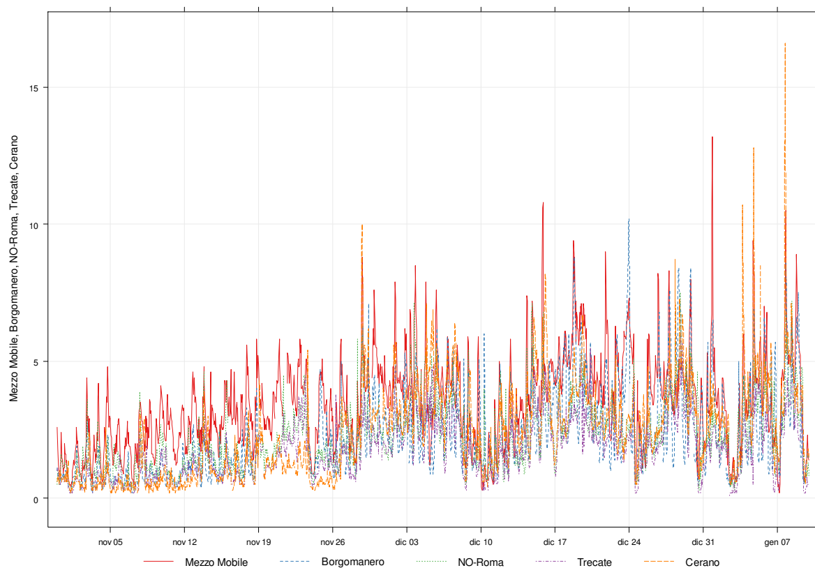
Figura 41: confronto delle medie orarie di Benzene
