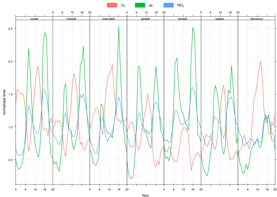
Figura 32: andamento medio orario in relazione al giorno della settimana – Confronto Ozono,
