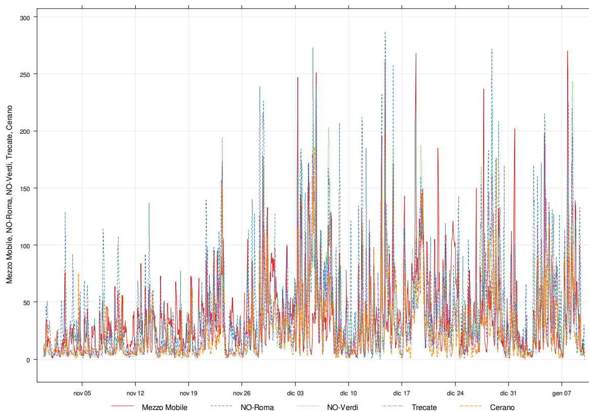
Figura 20: confronto delle medie orarie di Monossido di Azoto
