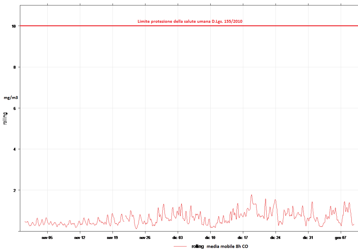
Figura 36: media mobile otto ore Monossido di Carbonio
