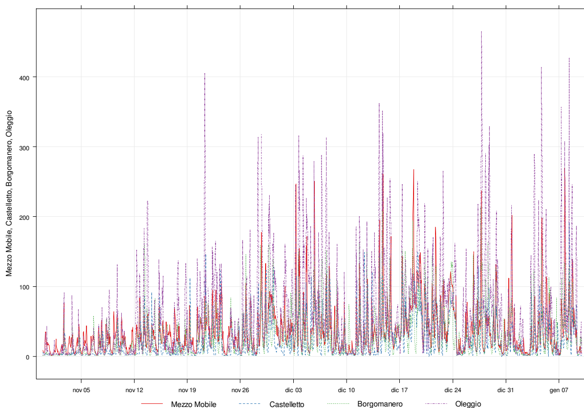
Figura 19: confronto delle medie orarie di Monossido di Azoto
