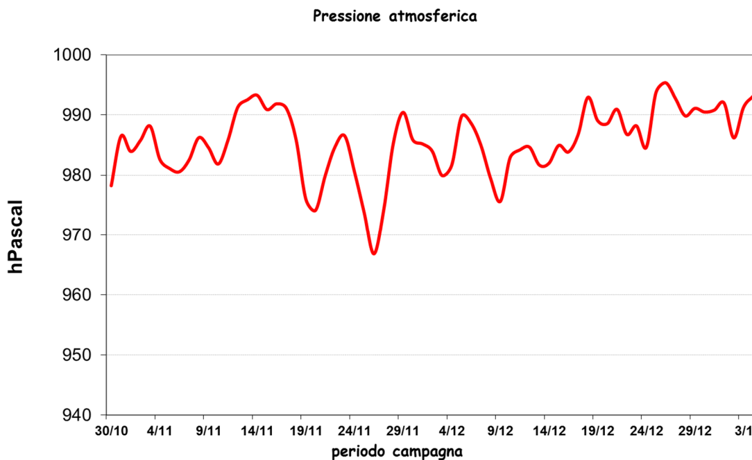
Figura 58: Pressione atmosferica media nel periodo
