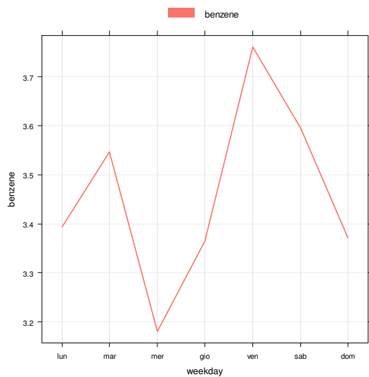
Figura 43: settimana tipo – Benzene
