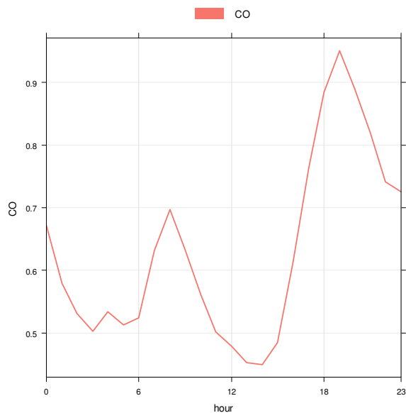
Figura 38: giorno tipo - Monossido di Carbonio
