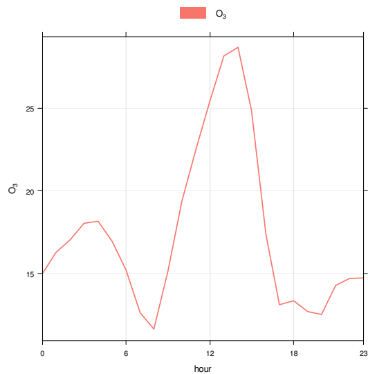
Figura 30: giorno tipo – Ozono
